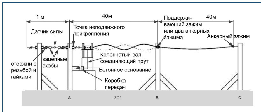
Рис. 3. Схема вибрационных испытаний
