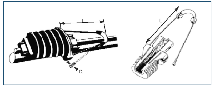
Рис. 1. Зажим «MALICRO»
