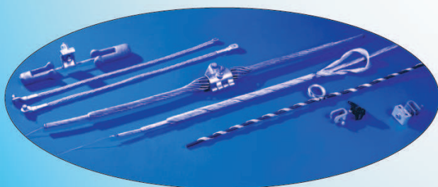
Крепления для кабеля типа ADSS и OPGW
